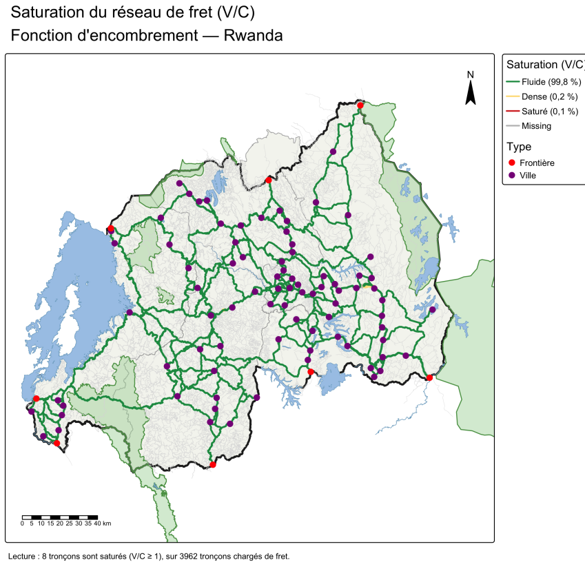
FIGURE 5.5 – Taux de saturation V/C du réseau — scénario de référence Source : auteur
