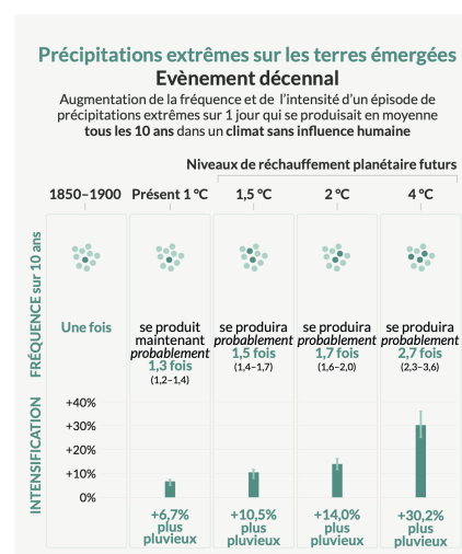
FIGURE 1.2 – Projection de l'évolution des précipitations extrêmes
